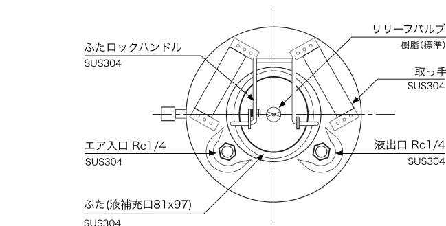
CT-N5シリーズ
