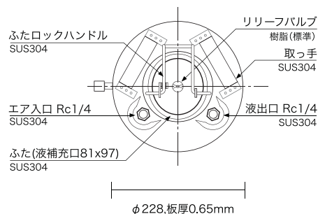
CT-N5 / CT-N10 / CT-N20 上部
